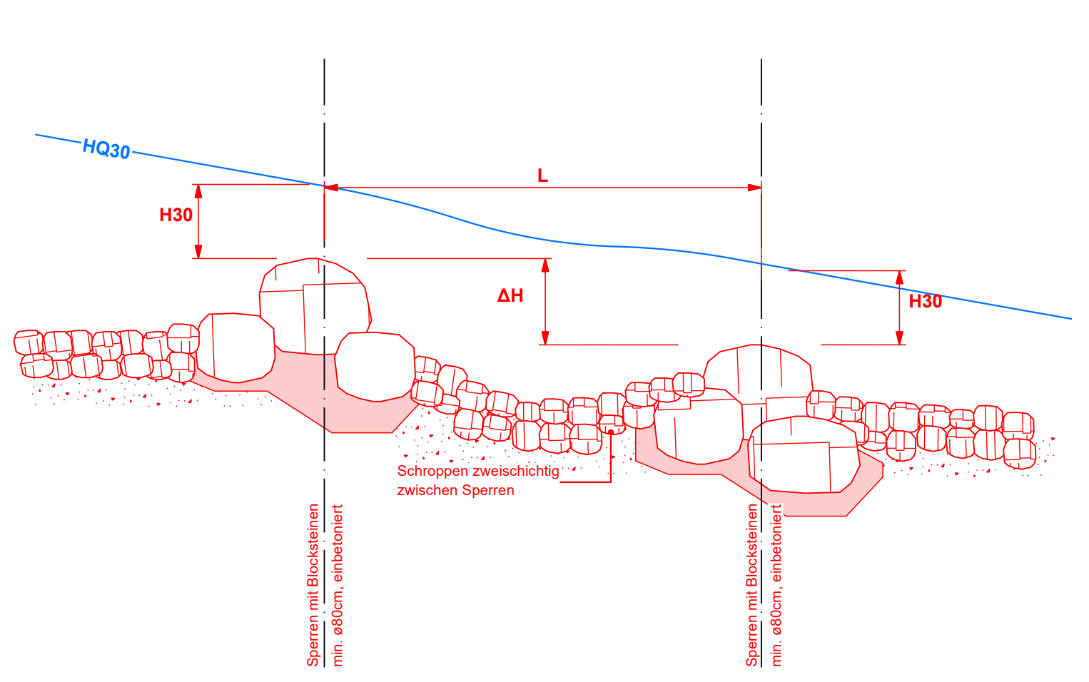
Systemschnitt 1:50 Gerinne mit Sperren
