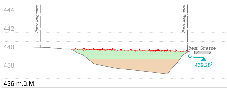
Querprofil C - C, 1:200
