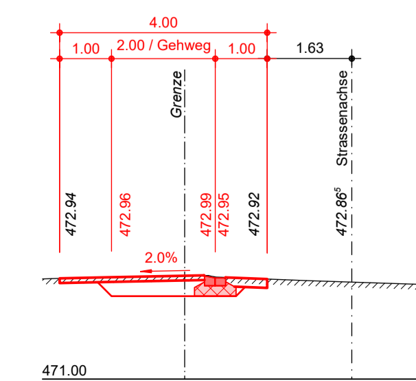
Querprofil 15, 1:100 (140.00 m)
