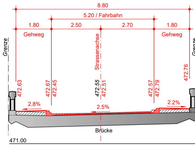
Querprofil 2, 1:100 (010.00 m)
