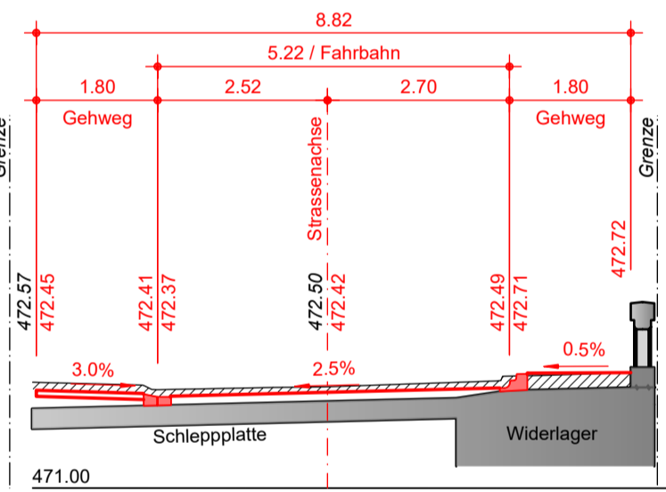
Querprofil 1, 1:100 (000.00 m)
