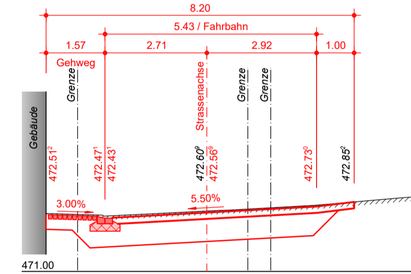
Querprofil 7, 1:100 (060.00 m)
