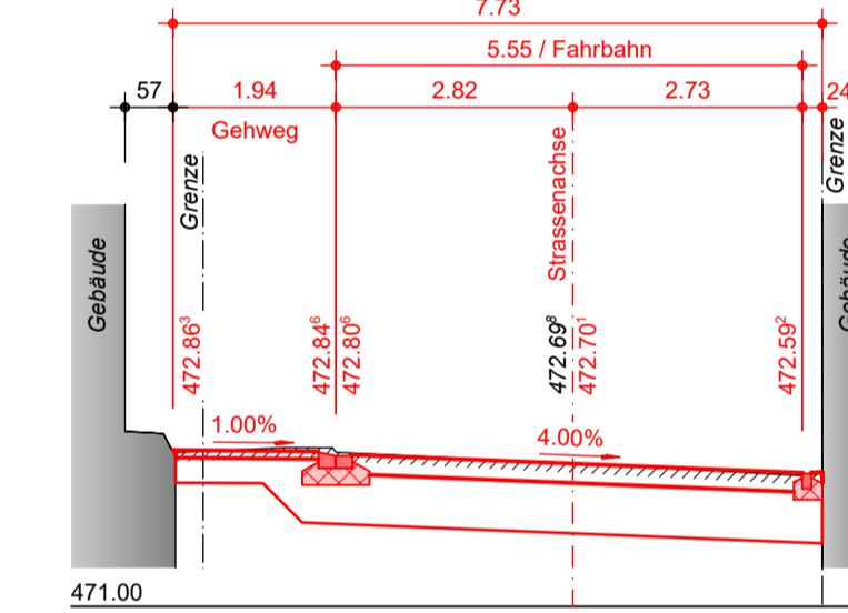
Querprofil 13, 1:100 (120.00 m)
