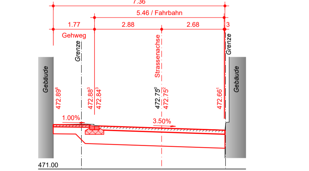
Querprofil 11, 1:100 (100.00 m)
