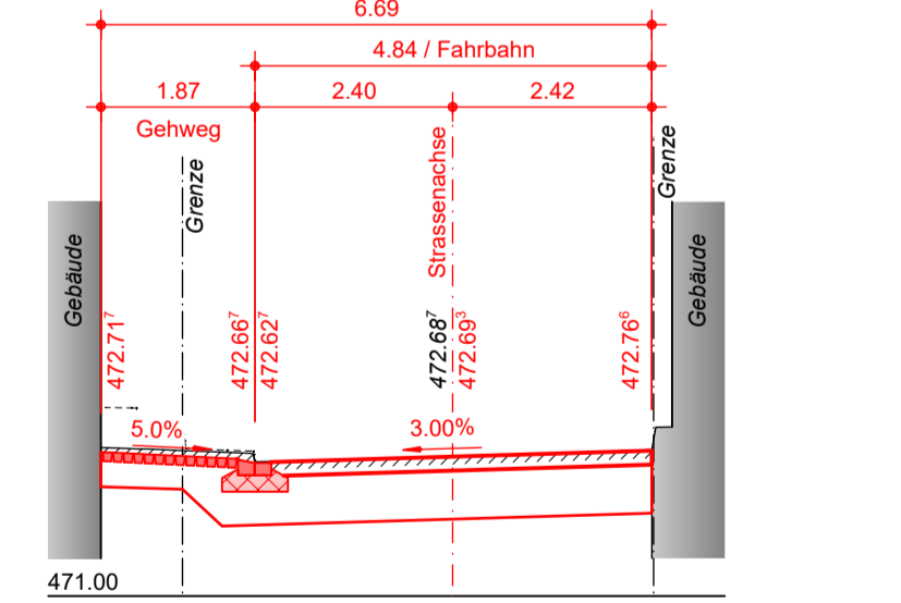
Querprofil 8, 1:100 (070.00 m)
