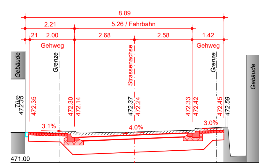
Querprofil 3, 1:100 (020.00 m)
