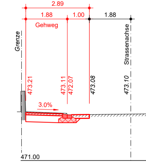
Querprofil 17, 1:100 (160.00 m)
