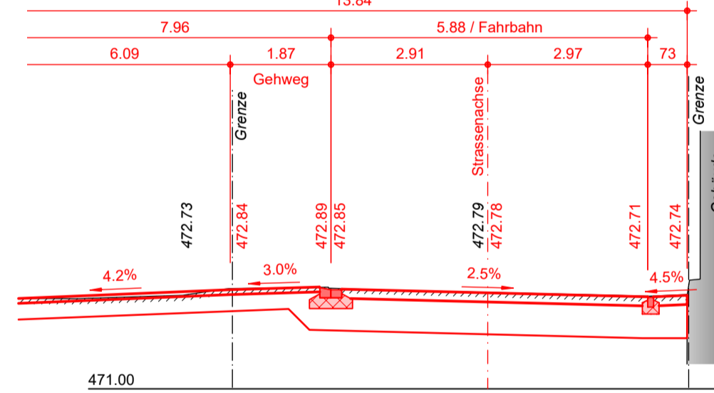
Querprofil 10, 1:100 (090.00 m)
