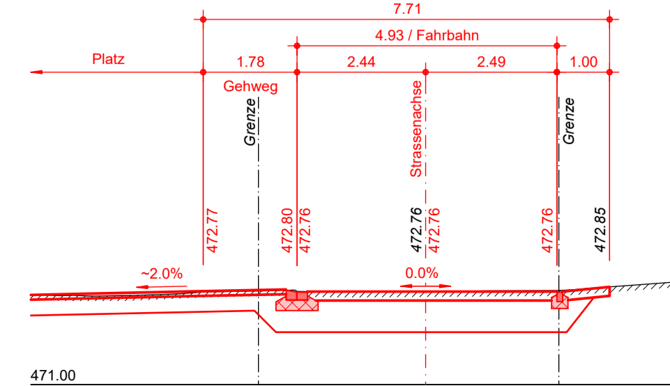
Querprofil 9, 1:100 (080.00 m)
