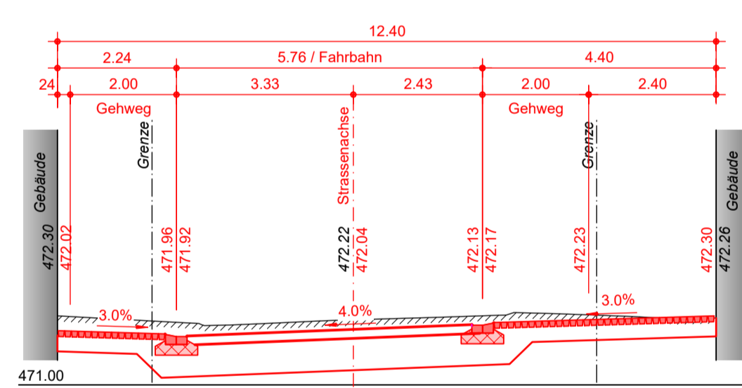
Querprofil 4, 1:100 (030.00 m)
