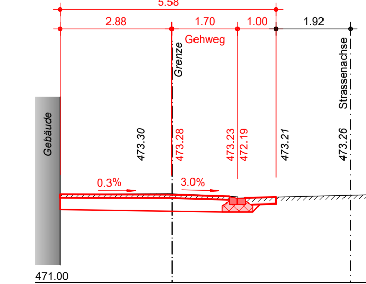
Querprofil 18, 1:100 (170.00 m)
