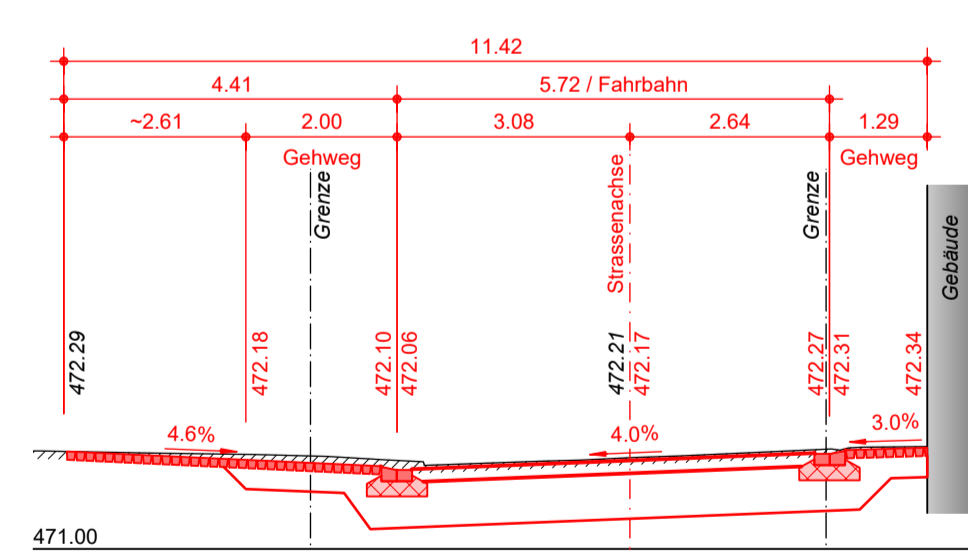
Querprofil 5, 1:100 (040.00 m)
