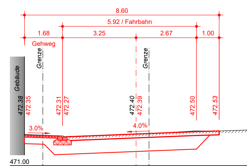
Querprofil 6, 1:100 (050.00 m)
