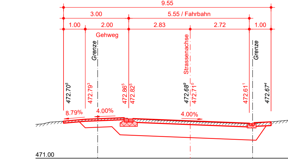
Querprofil 12, 1:100 (110.00 m)
