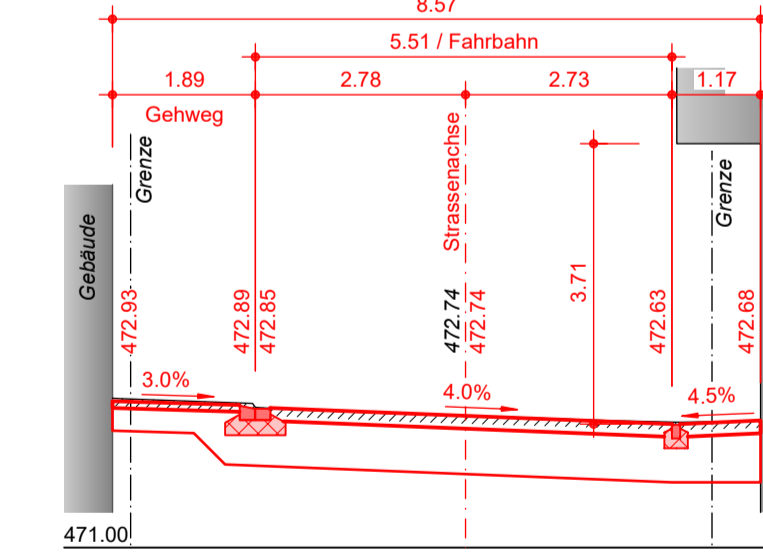
Querprofil 14, 1:100 (130.00 m)
